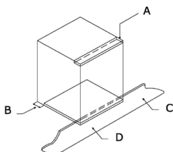
Fig. 7: Requisitos de ventilação e recorte para a instalação de um forno eléctrico simples numa unidade de cozinha standard. Requisitos de ventilação mínimos para as estantes superiores, de base e de suporte da parte traseira da unidade.
